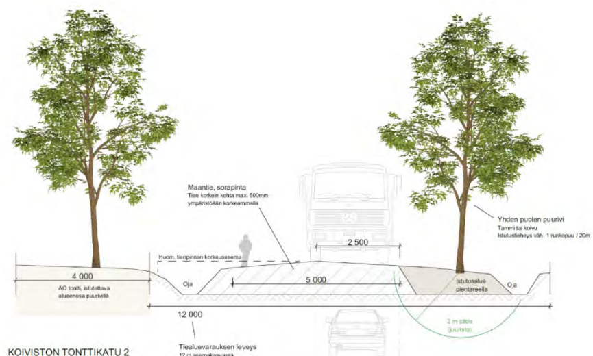
Kuva 46. Luonnos tonttikadun tieprofiilista.
