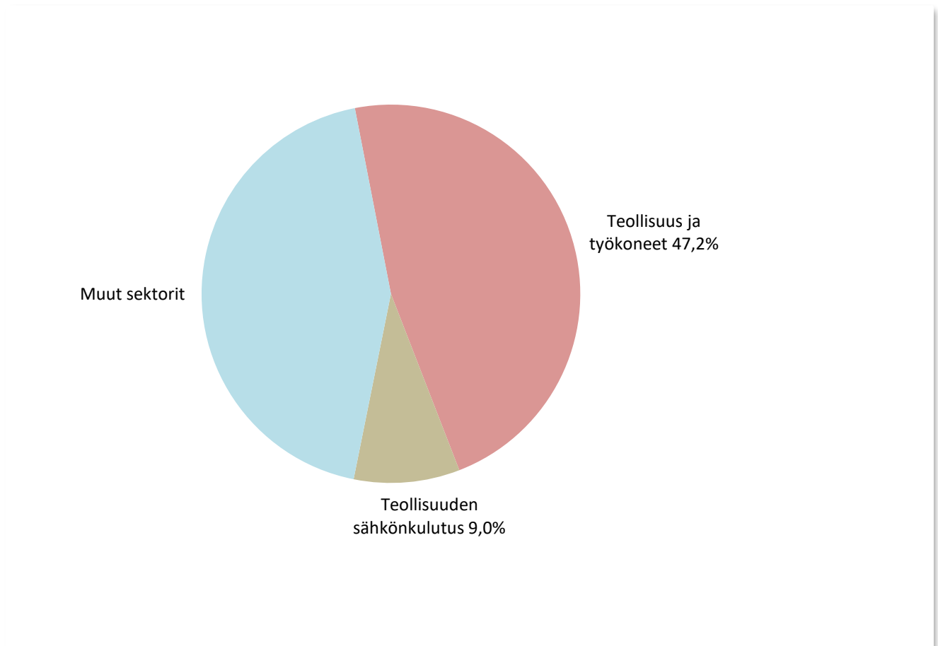
Kuva 7. Teollisuuden päästöjen osuus kokonaispäästöistä Äänekoskella vuonna 2016 ja sektorin jakautuminen eri päästölähteisiin.
