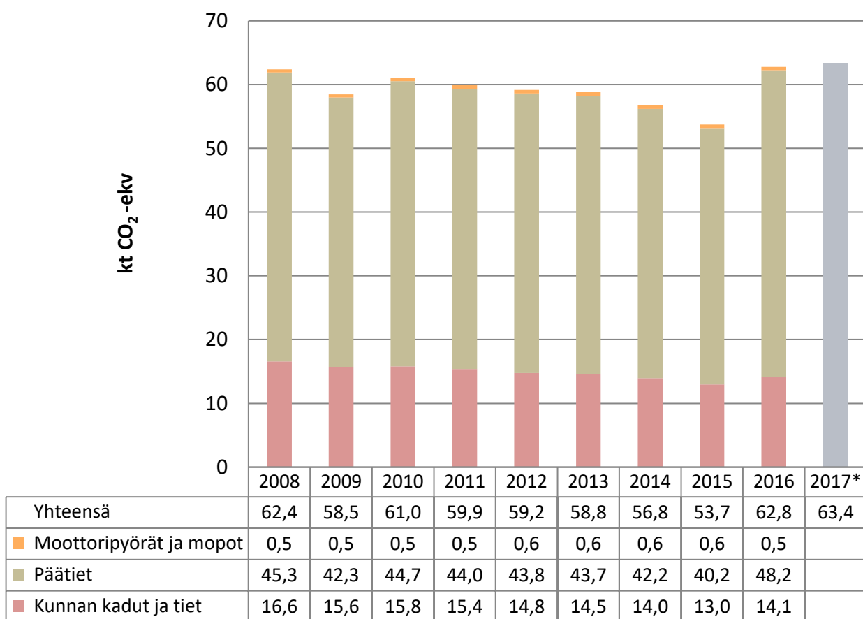
Kuva 10. Tieliikenteen päästöt Äänekoskella vuosina 2008–2017. Vuoden 2017 tieto on ennakkotieto, joka perustuu liikennemäärien muutoksiin kunnan alueella.
