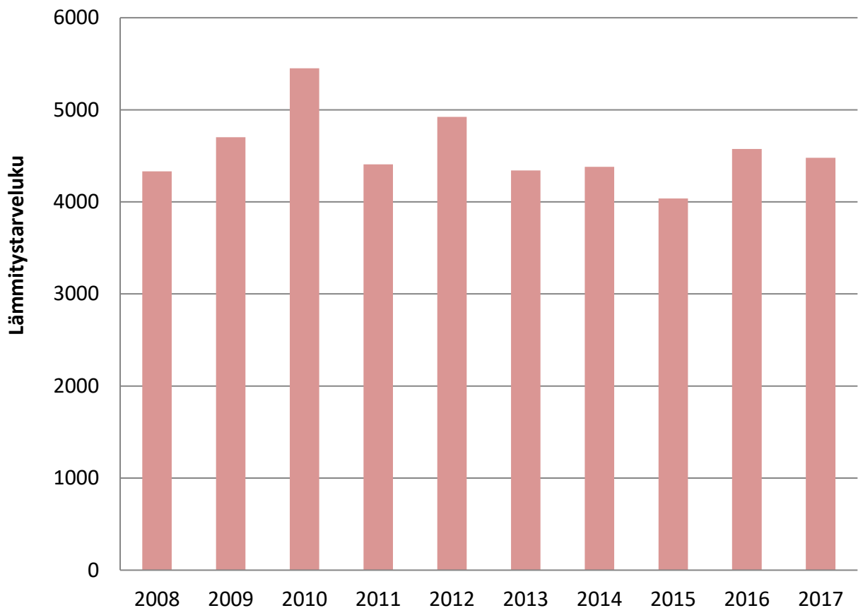
Kuva 4. Äänekosken lämmitystarveluvut vuosina 2008–2017.
