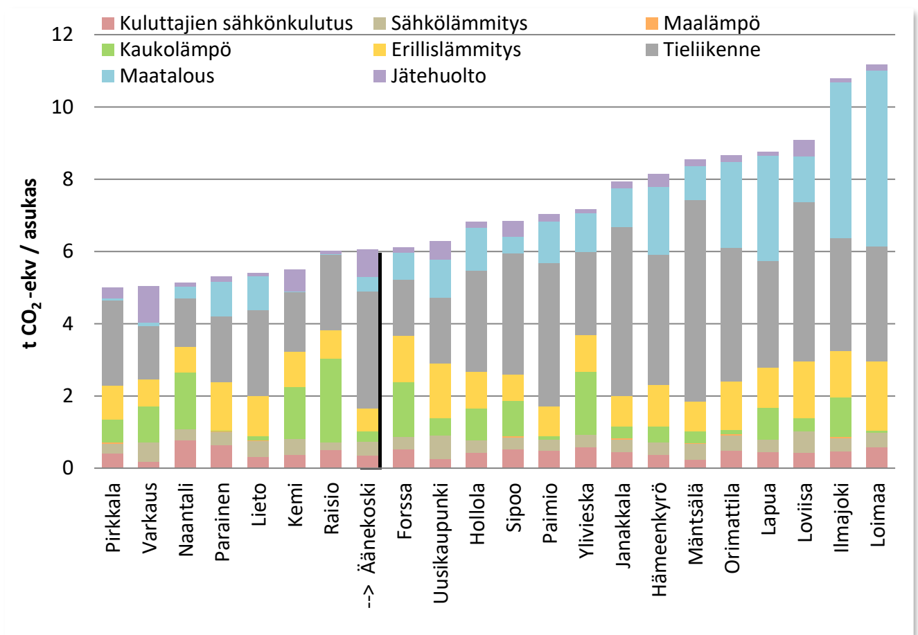
Kuva 22. CO 2 -raportissa mukana olevien 10000–25000 asukkaan kuntien asukaskohtaiset päästöt vuonna 2016 ilman teollisuutta.
