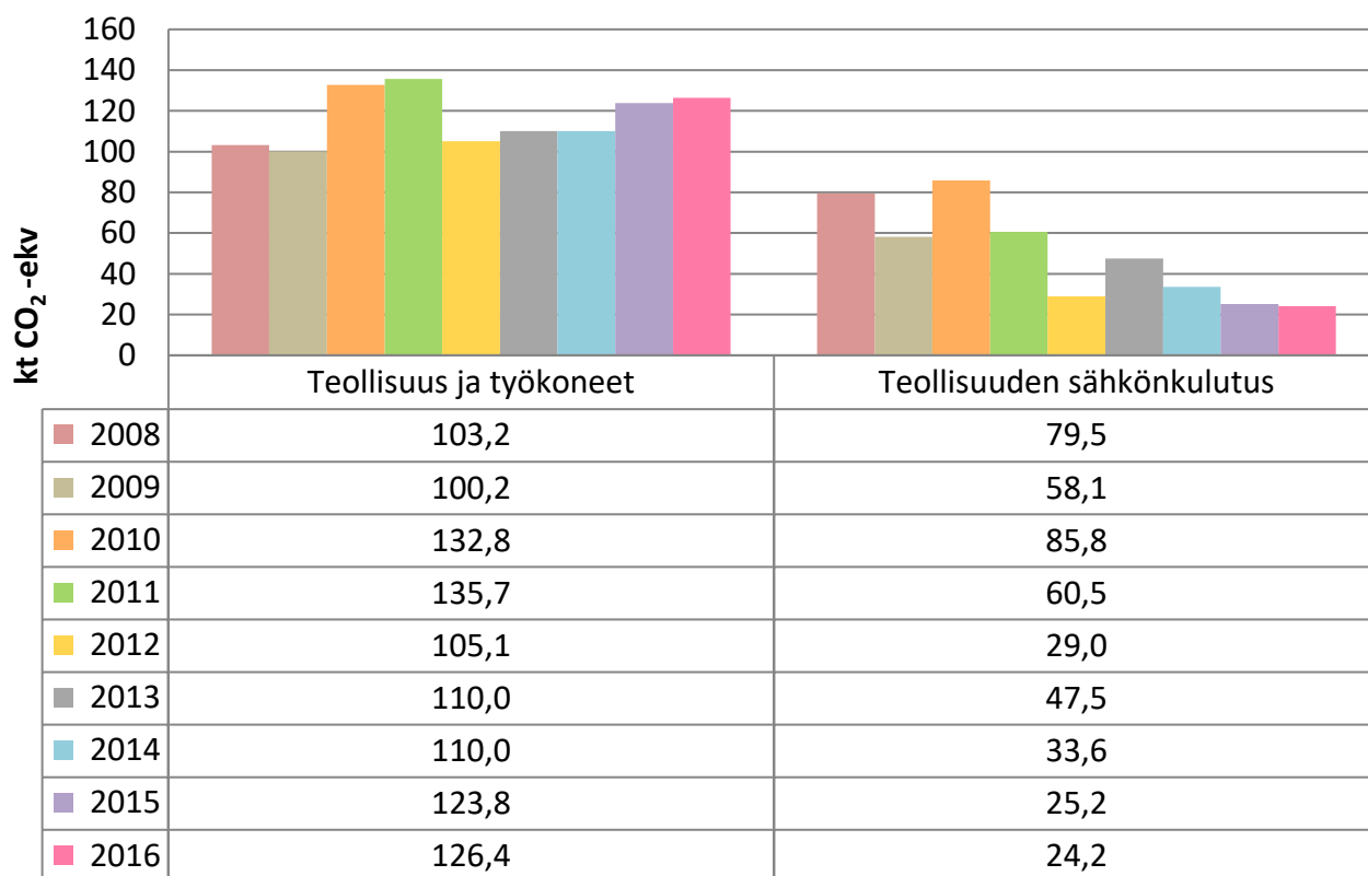
Kuva 8. Teollisuuden ja työkoneiden sekä teollisuuden sähkönkulutuksen päästöjen kehitys Äänekoskella vuosina 2008–2016.
