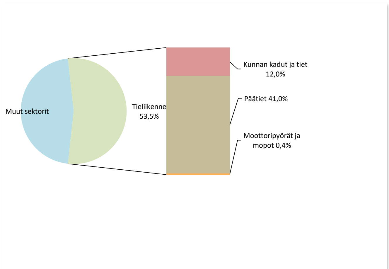
Kuva 9. Tieliikenteen päästöjen osuus kokonaispäästöistä (ilman teollisuutta) Äänekoskella vuonna 2016 ja sektorin jakautuminen eri päästölähteisiin.
