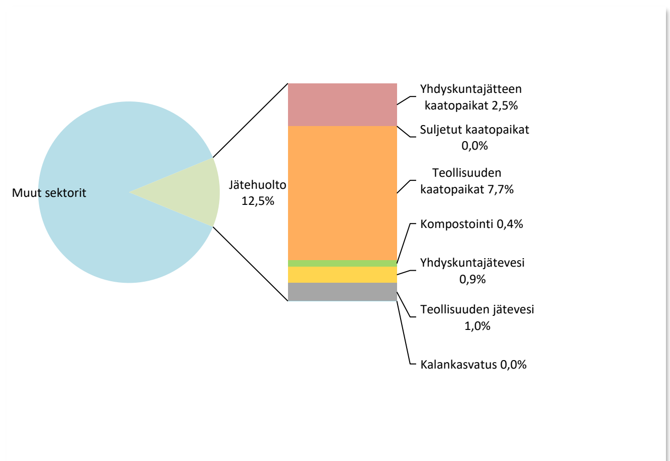
Kuva 13. Jätehuollon päästöjen osuus kokonaispäästöistä (ilman teollisuutta) Äänekoskella vuonna 2016 ja sektorin jakautuminen eri päästölähteisiin.
