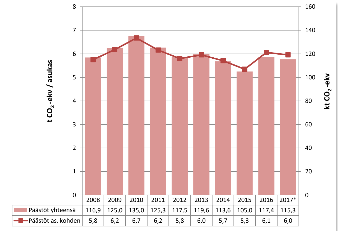
Kuva 18. Päästöt yhteensä ja asukasta kohden Äänekoskella vuosina 2008–2017 ilman teollisuutta. Vuoden 2017 tieto on ennakkotieto.
