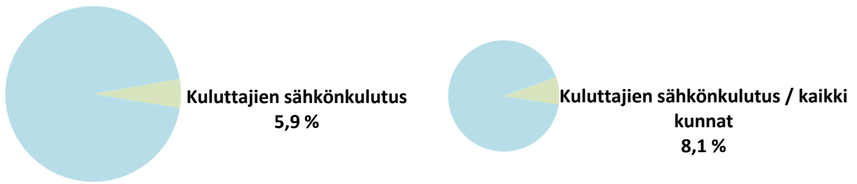
Kuva 2. Kuluttajien sähkönkulutuksen päästöjen osuus kokonaispäästöistä (ilman teollisuutta) Äänekoskella ja CO2-raportin kunnassa keskimäärin vuonna 2016.
