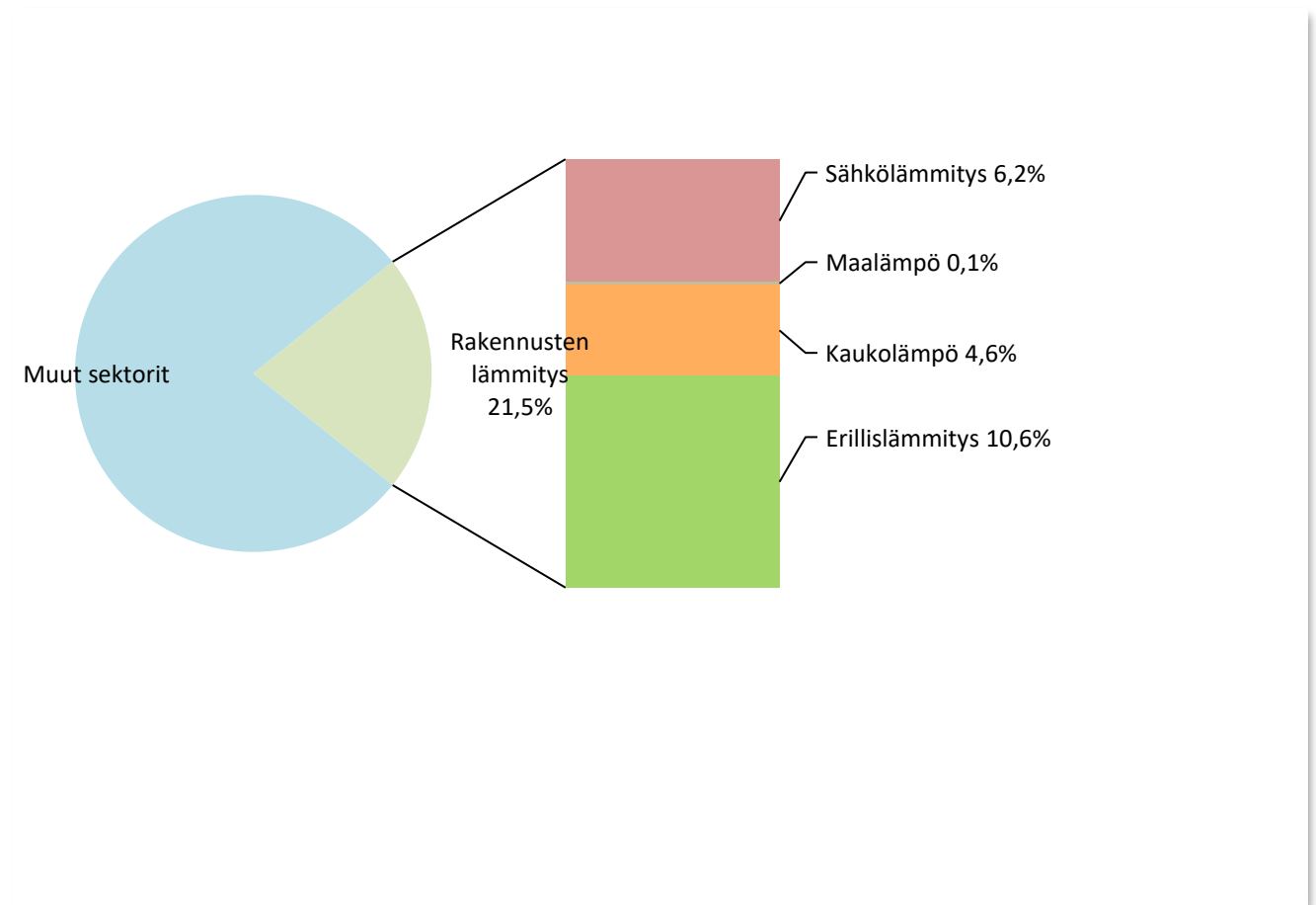
Kuva 5. Rakennusten lämmityksen päästöjen osuus kokonaispäästöistä (ilman teollisuutta) Äänekoskella vuonna 2016 ja sektorin jakautuminen eri päästölähteisiin.
