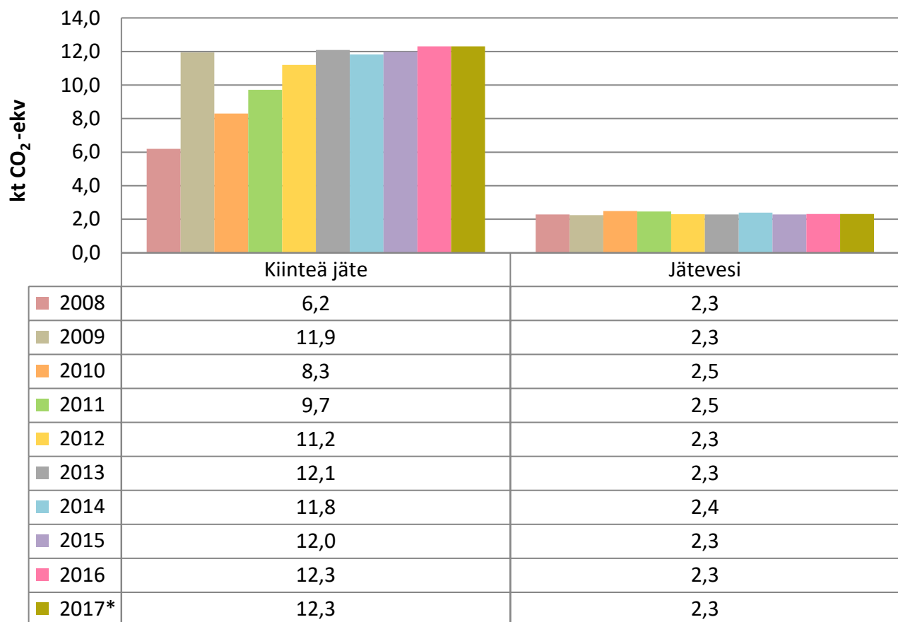
Kuva 14. Jätehuollon päästöjen kehitys Äänekoskella vuosina 2008–2017. Vuoden 2017 ennakkotietona on vuoden 2016 tieto.
