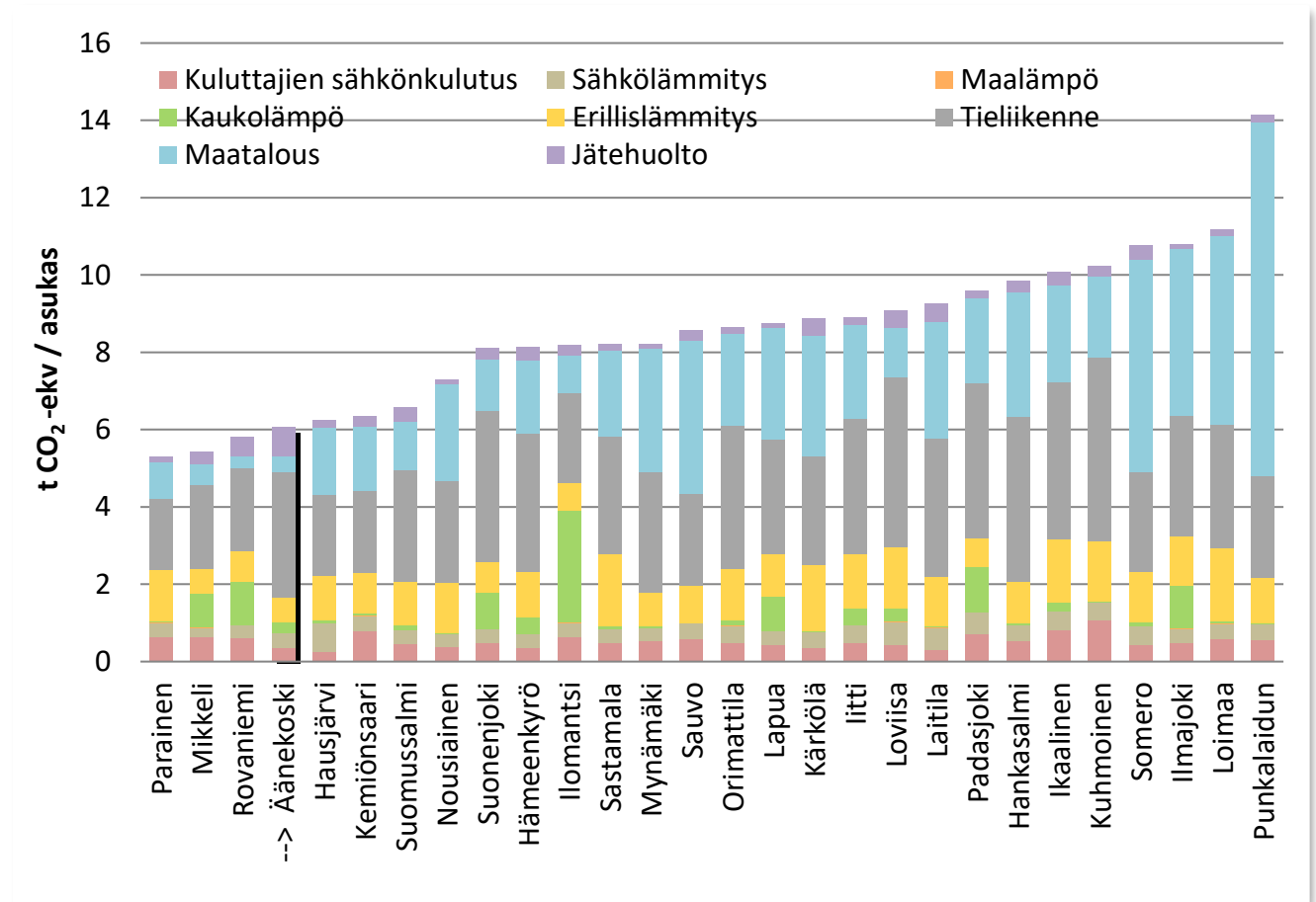
Kuva 23. Asukaskohtaisten päästöjen vertailu (ilman teollisuutta) vuonna 2016 sellaisissa CO2-raportin kunnissa, joissa on alle 25 asukasta maaneliökilometrillä.
