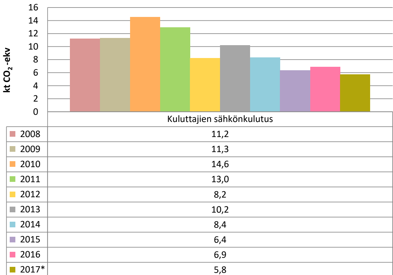
Kuva 3. Kuluttajien sähkönkulutuksen päästöjen kehitys Äänekoskella vuosina 2008–2017. Vuoden 2017 tieto on ennakkotieto.
