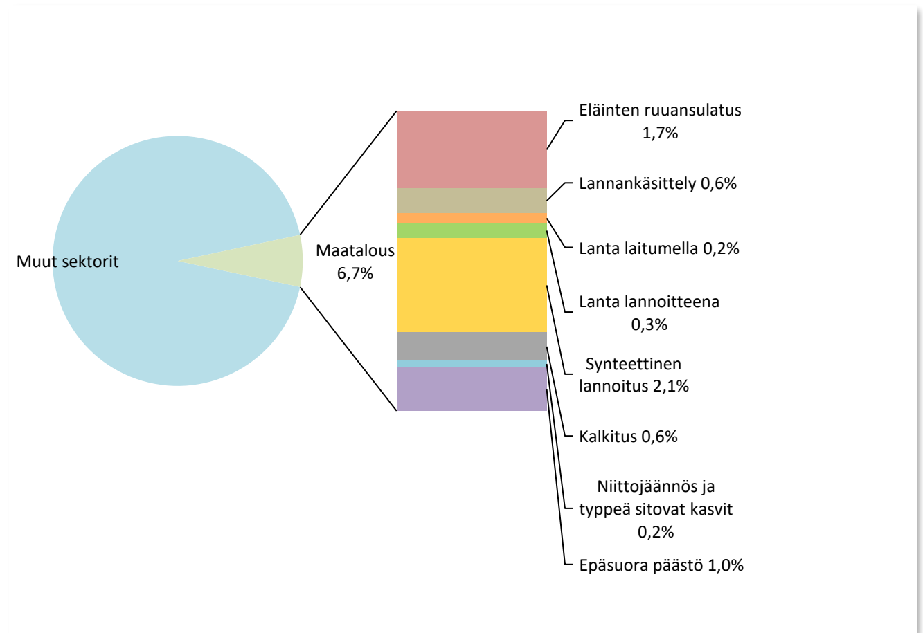
Kuva 11. Maatalouden päästöjen osuus kokonaispäästöistä (ilman teollisuutta) Äänekoskella vuonna 2016 ja sektorin jakautuminen eri päästölähteisiin.
