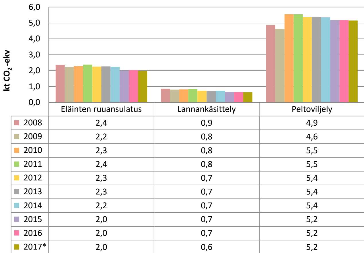
Kuva 12. Maatalouden päästöjen kehitys Äänekoskella vuosina 2008–2017 jaettuna eläinten ruuansulatuksen, lannankäsittelyn ja peltoviljelyn päästöihin.
