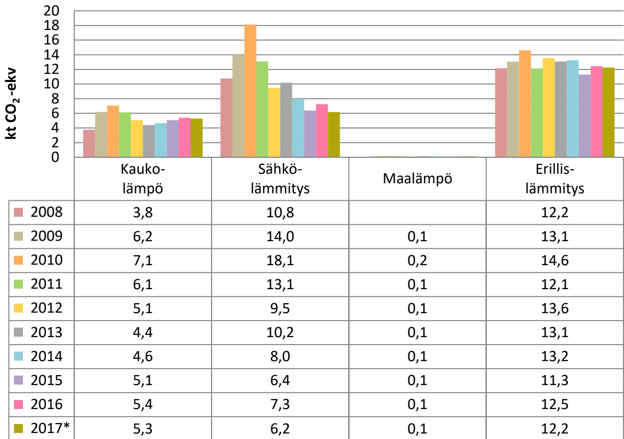
Kuva 6. Rakennusten lämmityksen päästöjen kehitys Äänekoskella vuosina 2008–2017. Vuoden 2017 tieto on ennakkotieto.
