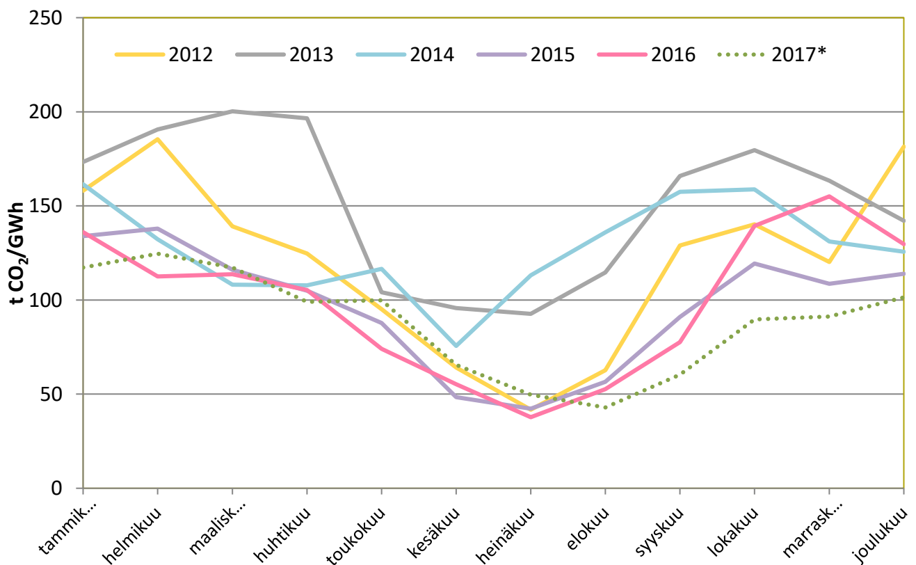
Kuva 1. Sähkönkulutuksen päästökerroin kuukausitasolla vuosina 2012–2017, laskettuna hyödynjakomenetelmällä Energiateollisuus ry:n aineistosta. Vuoden 2017 tieto on ennakkotieto.
