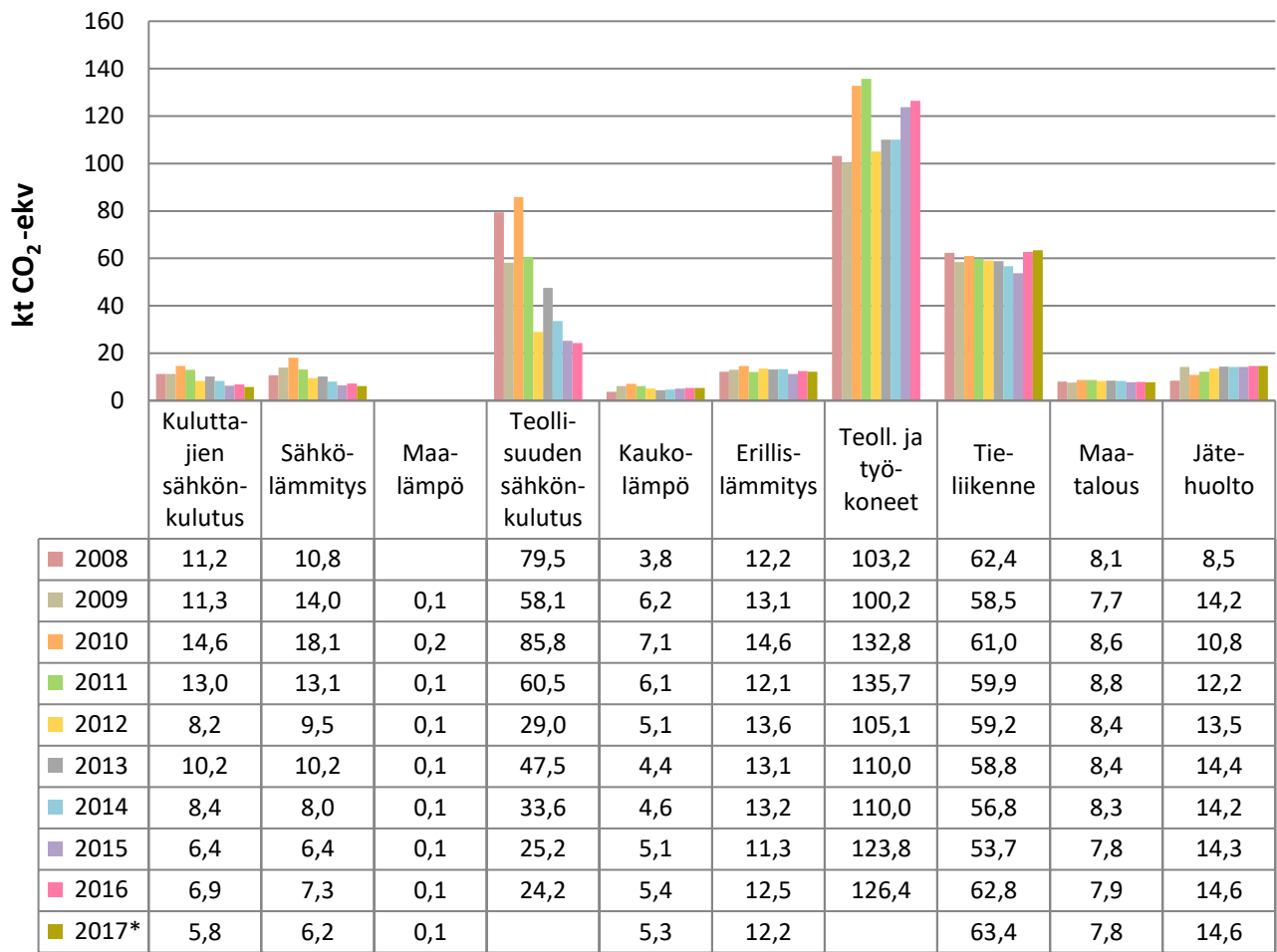
Kuva 17. Päästöt sektoreittain Äänekoskella vuosina 2008–2017. Vuoden 2017 tieto on ennakkotieto. Teollisuuden päästöille ei ole esitetty ennakkotietoa.
