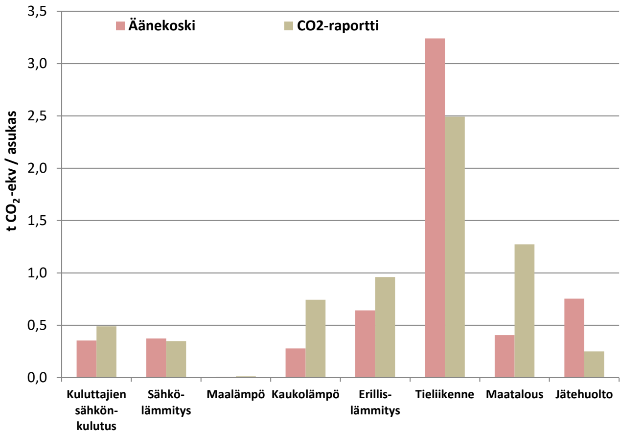
Kuva 20. Asukaskohtaisten päästöjen vertailu keskimääräiseen CO 2 -raportin kuntaan vuonna 2016.
