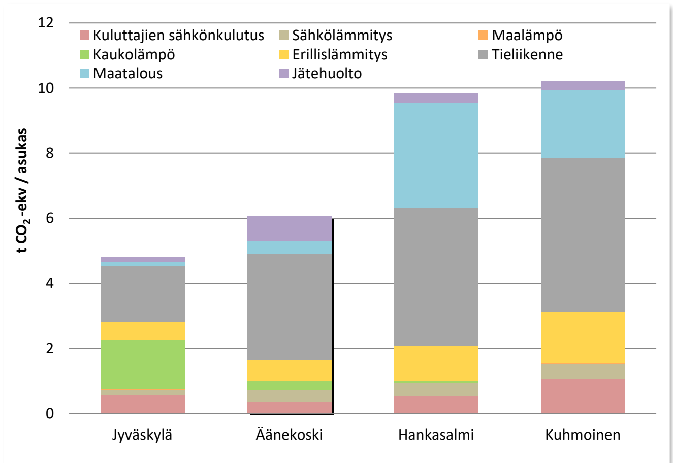
Kuva 21. CO 2 -raportissa mukana olevien Keski-Suomen kuntien asukaskohtaiset päästöt vuonna 2016 ilman teollisuutta.
