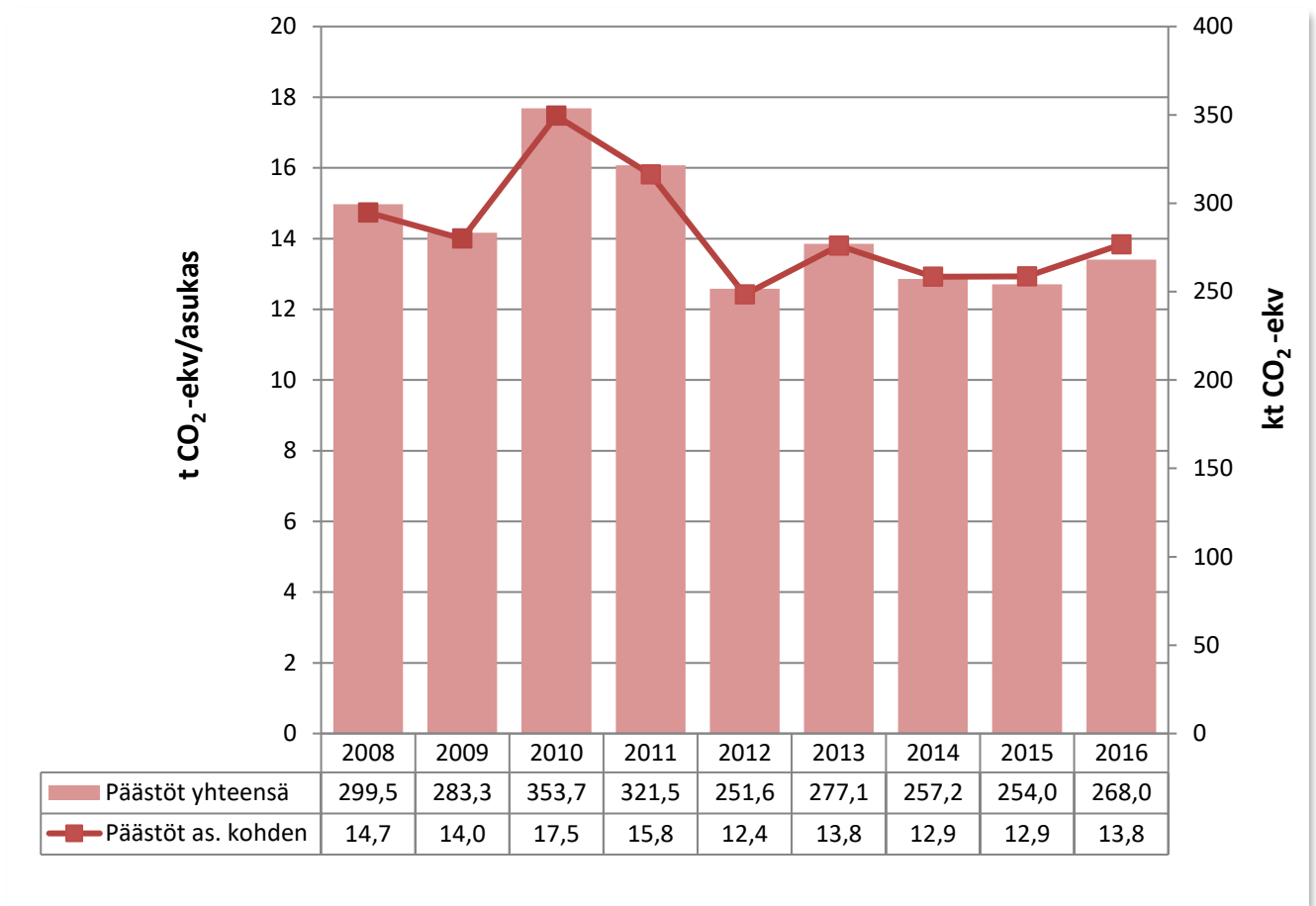
Kuva 19. Päästöt yhteensä ja asukasta kohden Äänekoskella vuosina 2008–2016, kun teollisuuden päästöt ovat mukana tarkastelussa.
