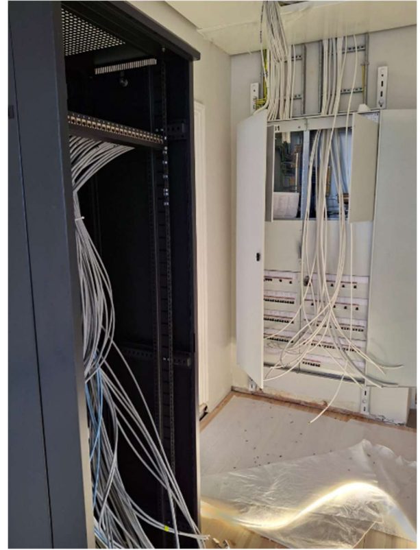
Kaapeleita on vedetty sähkö- ja ATK-keskuksille.
