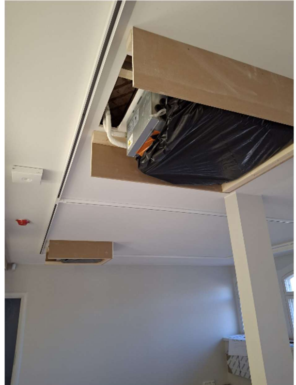
Jäähdytyksen sisäyksiköt koteloidaan piiloon kipsilevyllä. Kotelon alalaitaan tulee jäähdytyslaitteen oma ritilä ja etulaitaan huoltoluukku.
